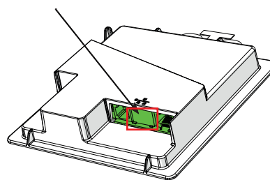
Ethernet anslutningsport (Modbus TCP/IP)
